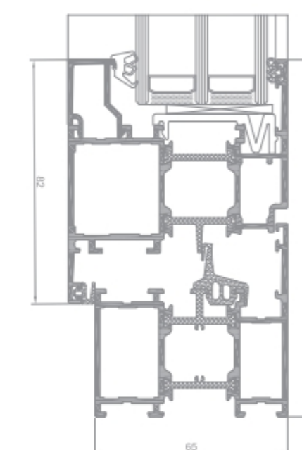
řez oknem IP
