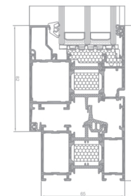
řez oknem IP i+
