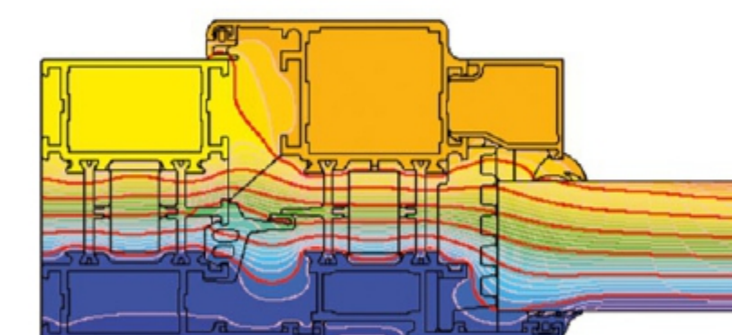
příklad rozložení izoterm v sestavě rámu a okenního křídla IP i+ (IP O11 + IP O21)
